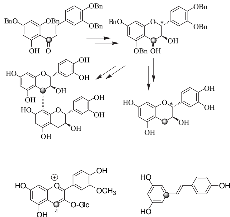
Fig. 3 : Préparation de polyphénols marqués au ^{13}\text{C}
